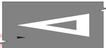
R5 - Marca de cedência de prioridade
